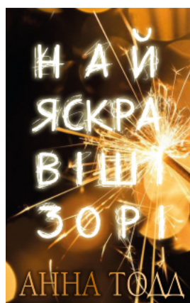
Найяскравіші зорі
